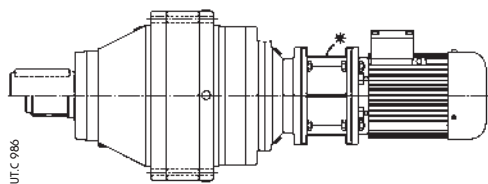
MLS / MLA montaggio tra riduttore e motore o motorvariante mounted between gear reducer and motor or motor-variator
